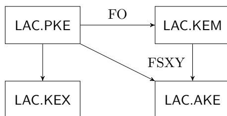
图 1. 基于格的密码系统LAC
